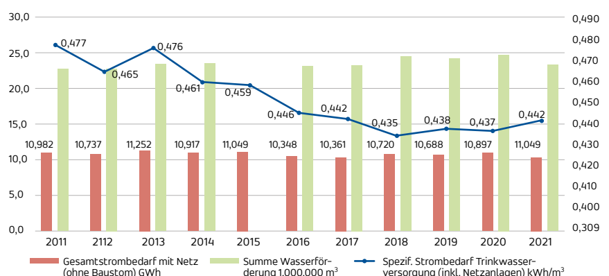
Gesamtstrombedarf Bereich Trinkwasser absolut und spezifisch
