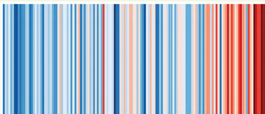
Warming Stripes Deutschland 1881-2020
