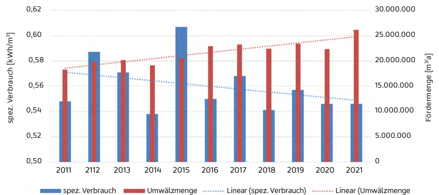
Spezifischer Verbrauch Heizwasserumwälzpumpen
